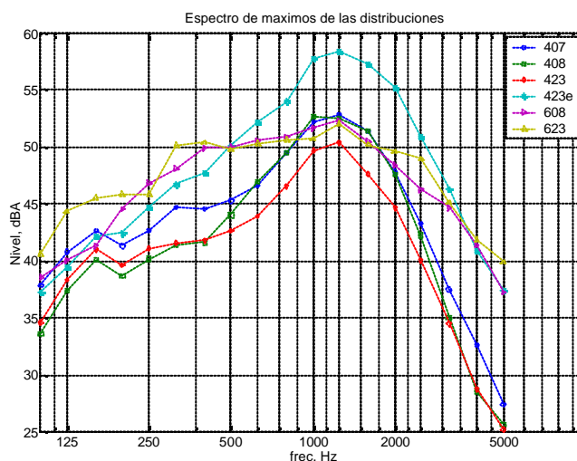
Figura 2. Espectro de máximos de las distribuciones de las medidas indicadas. El primer dígito indica el punto de medida (4 vivienda, 6 plataforma), los dos siguientes el día de medida, y la letra e que el micrófono se situó frente a la fachada del edificio)
