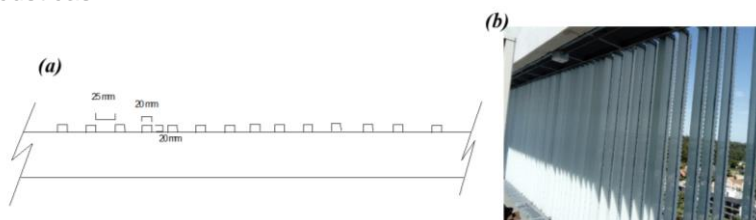
Ilustración 8. Generador de vorticidad propuesto, esquema (a) y fotografía una vez instalado (b)
