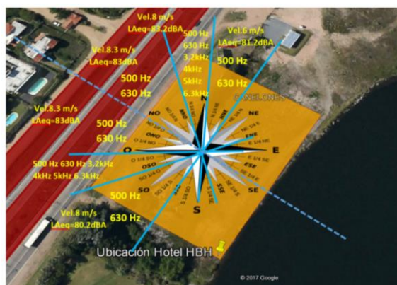
Ilustración 7 Frecuencias predominantes emitidas para diferentes condiciones de viento
