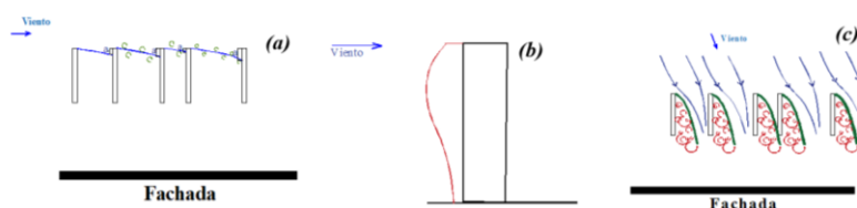
Ilustración 3. Flujo del viento paralelo a la fachada del edificio (a); Distribución de la presión del viento sobre la fachada de un edificio debido a la interacción con el viento (b); Flujo de viento perpendicular a la fachada del edificio (c).
