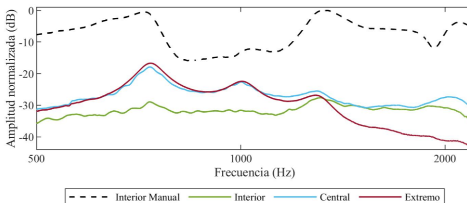
Figura 5 – Espectro obtenido de manera experimental. Métodos: Manual y Automáticos.
