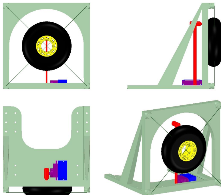
Figura 3 – Configuración experimental - Diseño Conceptual - Final - 5 Vertical. Se muestra en rojo el martillo excitador, en violeta el servomotor SG-90 y en azul el soporte de anclaje del servomotor a la estructura.
