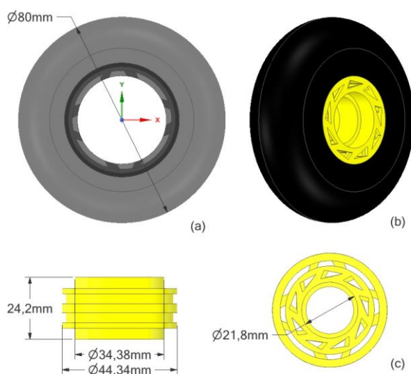
Figura 1 – Estructura de una rueda - UnderCover - 80 mm: Goma de la rueda (a), Rueda completa en perspectiva (b), Núcleo rígido de la rueda (c).
