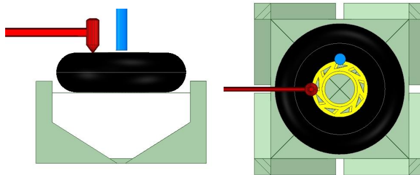
Figura 2 – Esquema de montaje experimental – Configuración manual - Instrumental de impacto marcado en Rojo – Instrumental de medida marcado en Azul – Soporte de medida en verde y gomas elásticas representadas como líneas.
