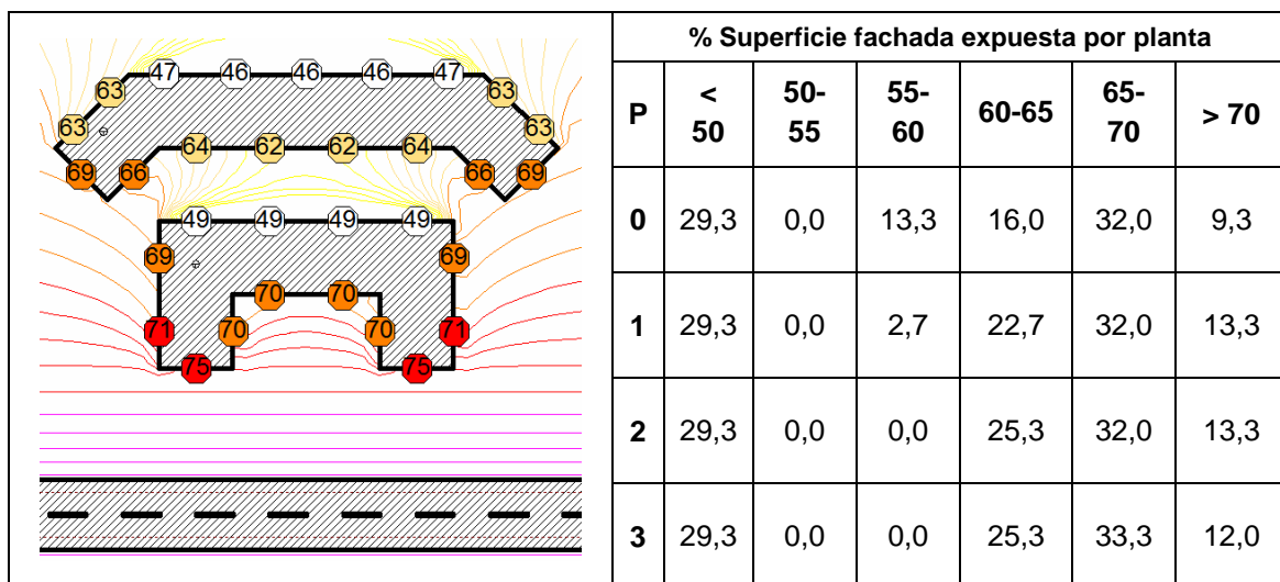
Figura 5: Porcentaje de superficie de fachada expuesta caso 3
