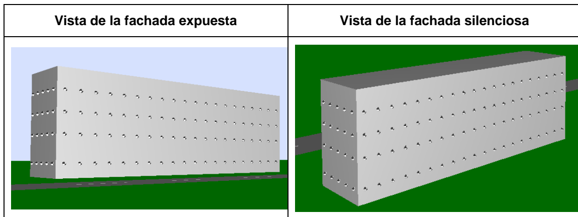
Figura 2. Matriz de receptores en fachada expuesta y silenciosa
