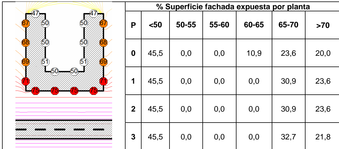
Figura 4: Porcentaje de superficie de fachada expuesta caso 2
