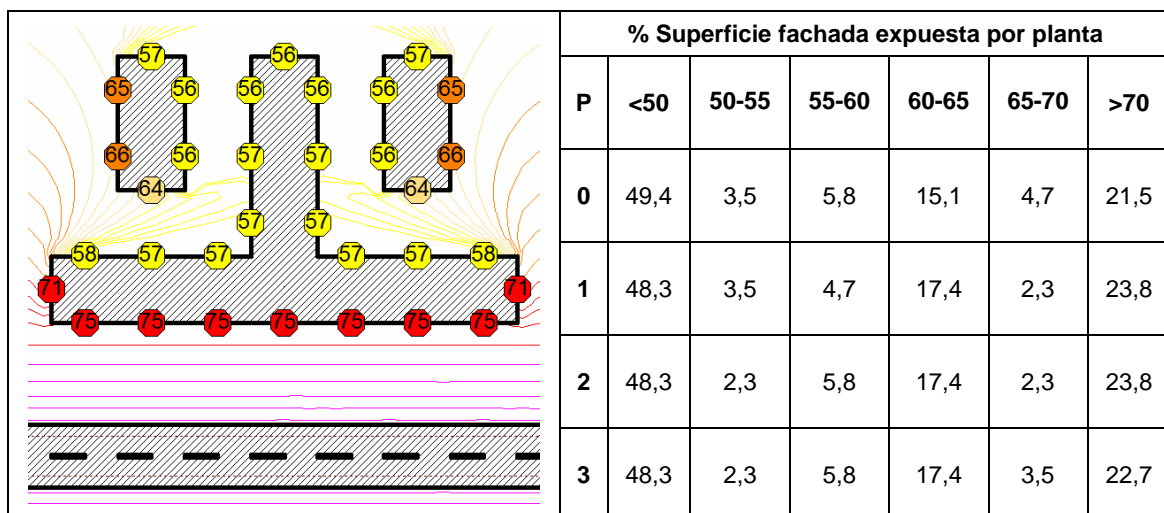
Figura 8: Porcentaje de superficie de fachada expuesta caso 6
