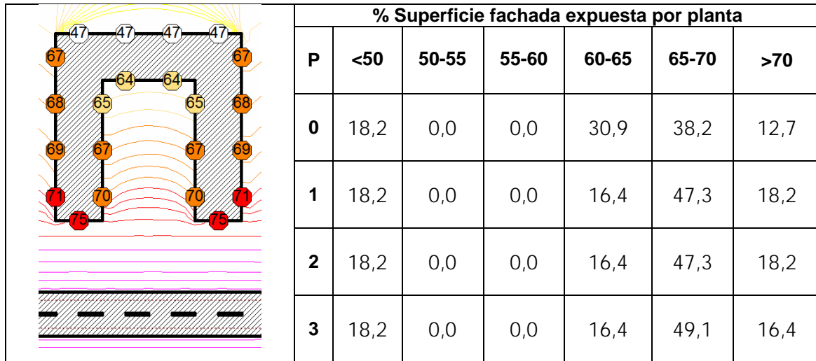
Figura 3: Porcentaje de superficie de fachada expuesta caso 1
