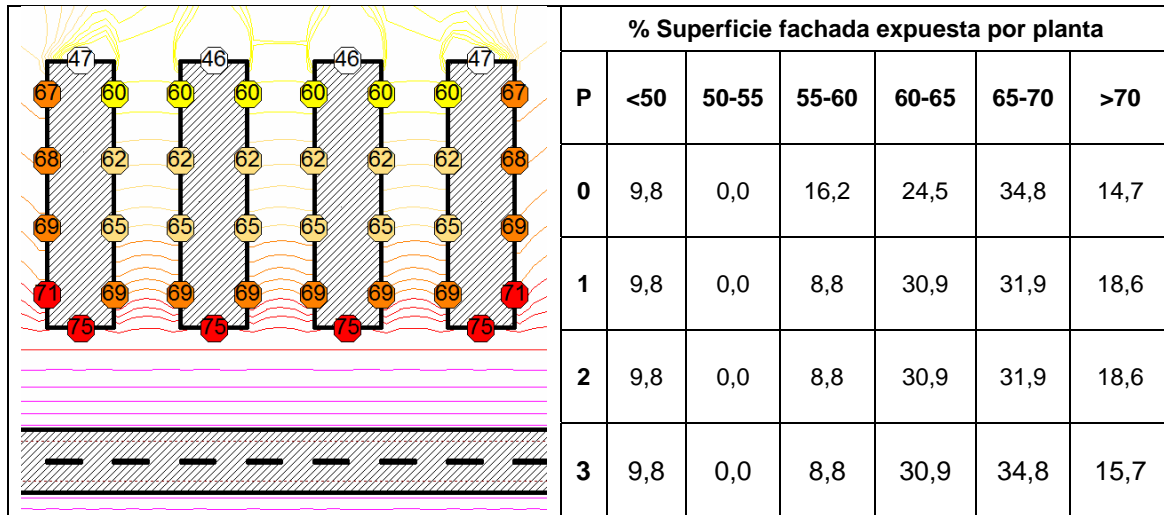
Figura 9: Porcentaje de superficie de fachada expuesta caso 7
