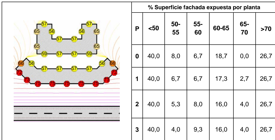
Figura 6: Porcentaje de superficie de fachada expuesta caso 4
