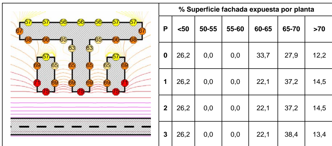
Figura 7: Porcentaje de superficie de fachada expuesta caso 5
