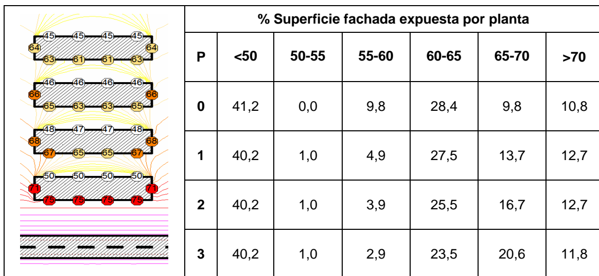
Figura 10: Porcentaje de superficie de fachada expuesta caso 8
