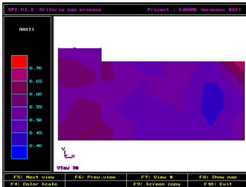
Figura 3: Distribución de SPL global y RASTI debidos a la fuente 'tutti'
