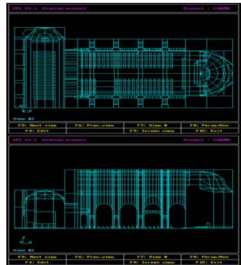
Figura 2b: Modelo de la iglesia
