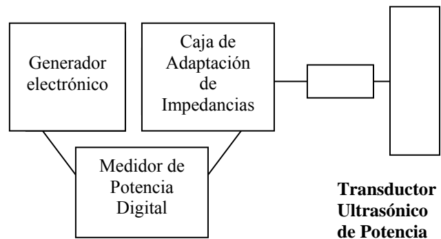
Figura 5. Esquema del sistema ultrasónico completo utilizado.
