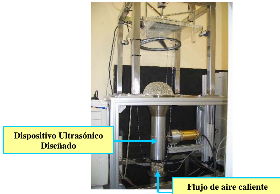
Figura 8. Sistema de secado por lecho fluido asistido por ultrasonidos de potencia.
