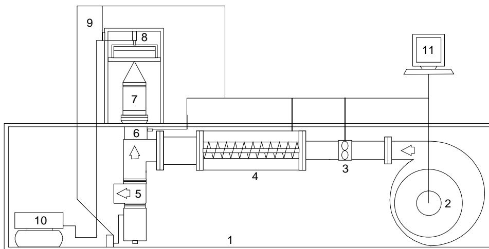
Figura 1. Esquema de un sistema de deshidratación por lecho fluido: 1 armazón; 2 ventilador; 3 anemómetro; 4 elementos calefactores; 5 válvula neumática; 6 control y medida de la temperatura, 7 recipiente de las muestras; 8 balanza; 9 elevador; 10 aire comprimido, 11 PC.
