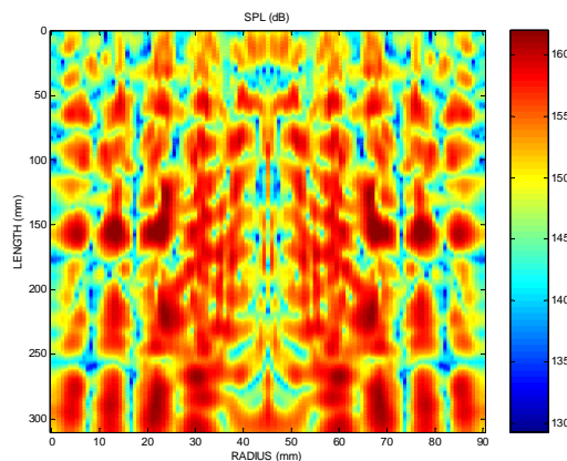
Figura 7. Distribución del campo acústico en el interior del cilindro vibrante cuando es excitado con una potencia = 75W
