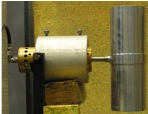
Figura 4. Dispositivo ultrasónico (transductor y vibrador) y soporte.
