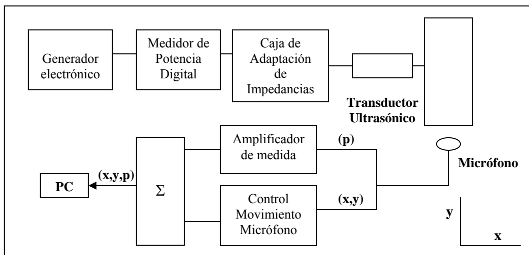
Figura 6. Esquema del dispositivo experimental utilizado y de los sistemas de control utilizados en el proceso de medida del campo acústico.
