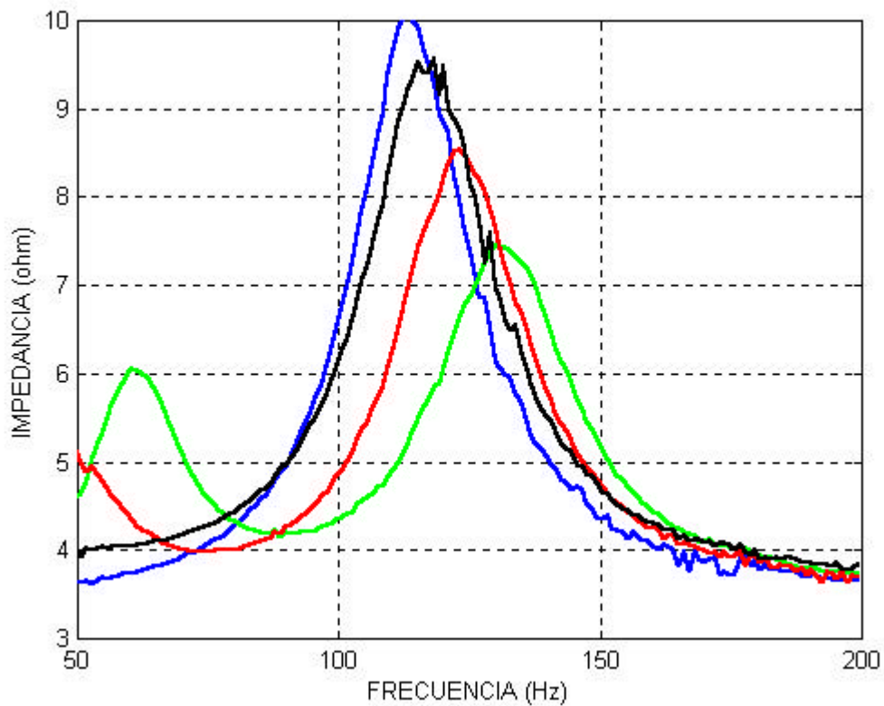
Figura 6. Impedancia del altavoz A2 en caja cerrada (azul), orificio (verde), tubo de 3 cm (rojo), y tubo de 10 cm (negro)
