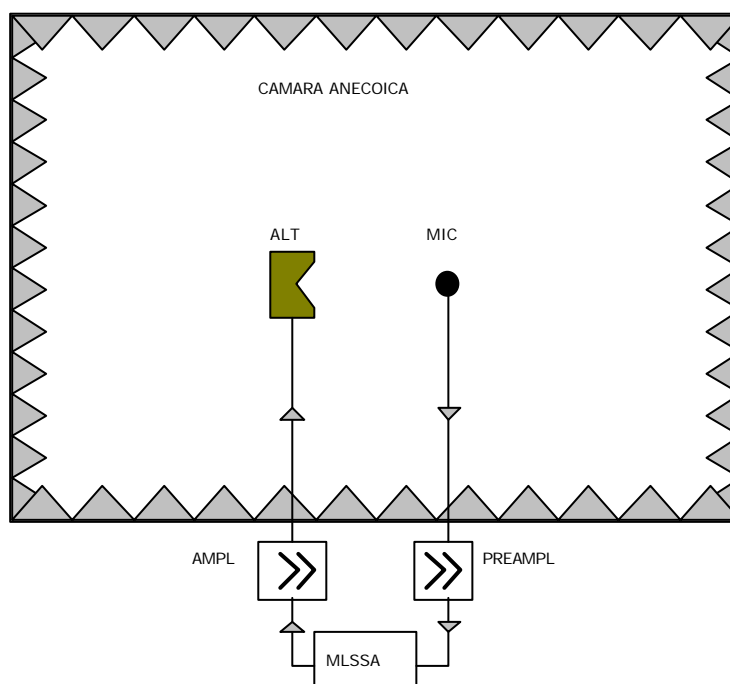
Figura 1. Esquema de la medida de altavoces en cámara anecoica con el sistema MLSSA
