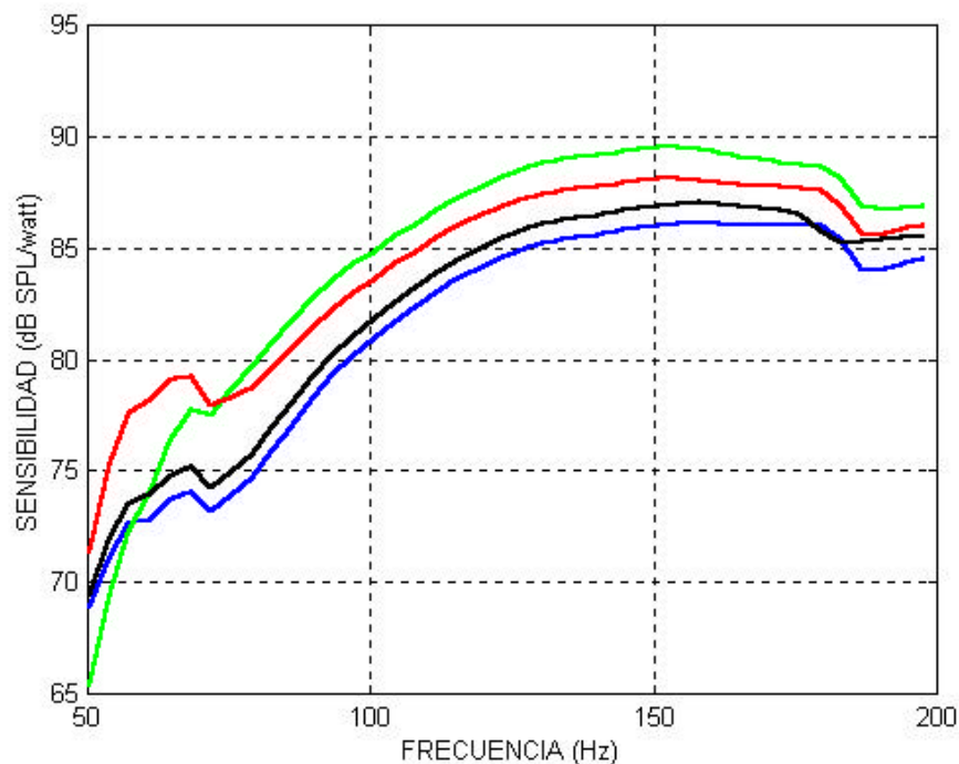
Figura 2. Sensibilidad del altavoz A1 en caja cerrada (azul), orificio (verde), tubo de 3 cm (rojo), y tubo de 10 cm (negro)
