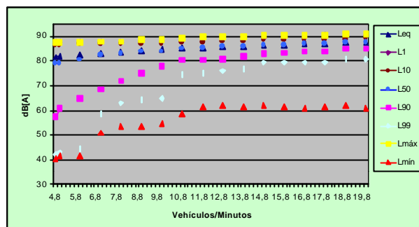
Figura 7. Zona con solapamiento de eventos
