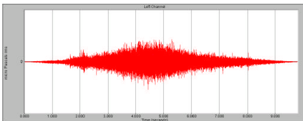
Figura 1. "Registro de pasaje base", correspondiente a la grabación real del pasaje de un vehículo aislado.
