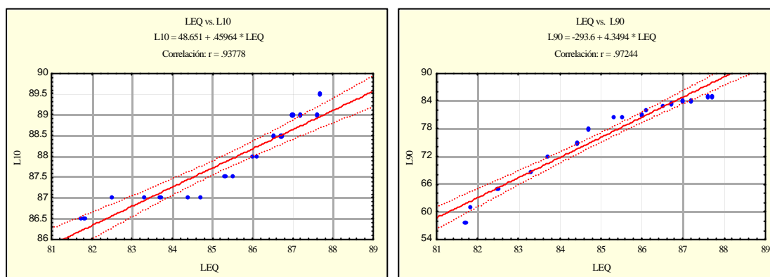
Figura 8. Correlación entre parámetros en la zona con solapamiento de eventos
