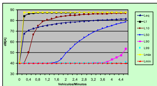
Figura 5. Zona sin solapamiento de eventos.
