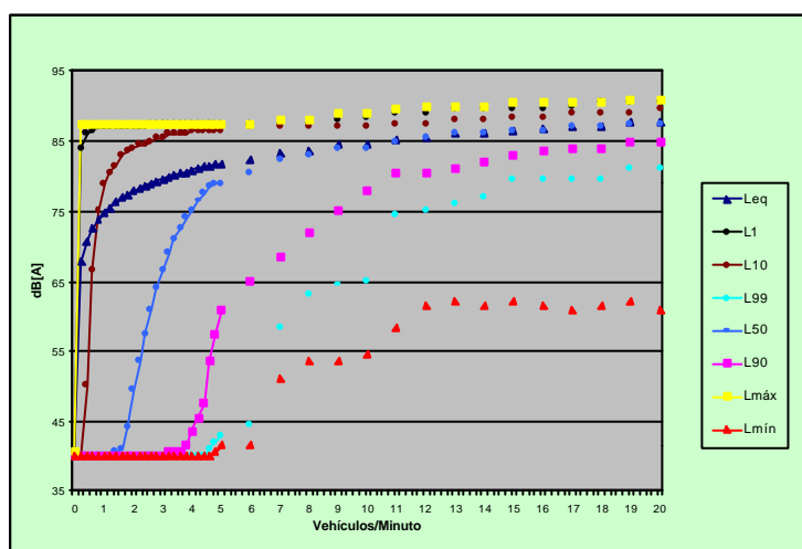
Figura 4. Variación de las parámetros estadísticos medidos en función de la densidad promedio de vehículos.
