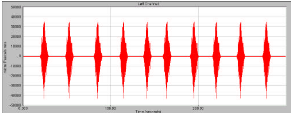
Figura 2. Registro de medición, correspondiente al pasaje de 10 vehículos en 5 minutos (densidad promedio = 2 vehículos por minuto)
